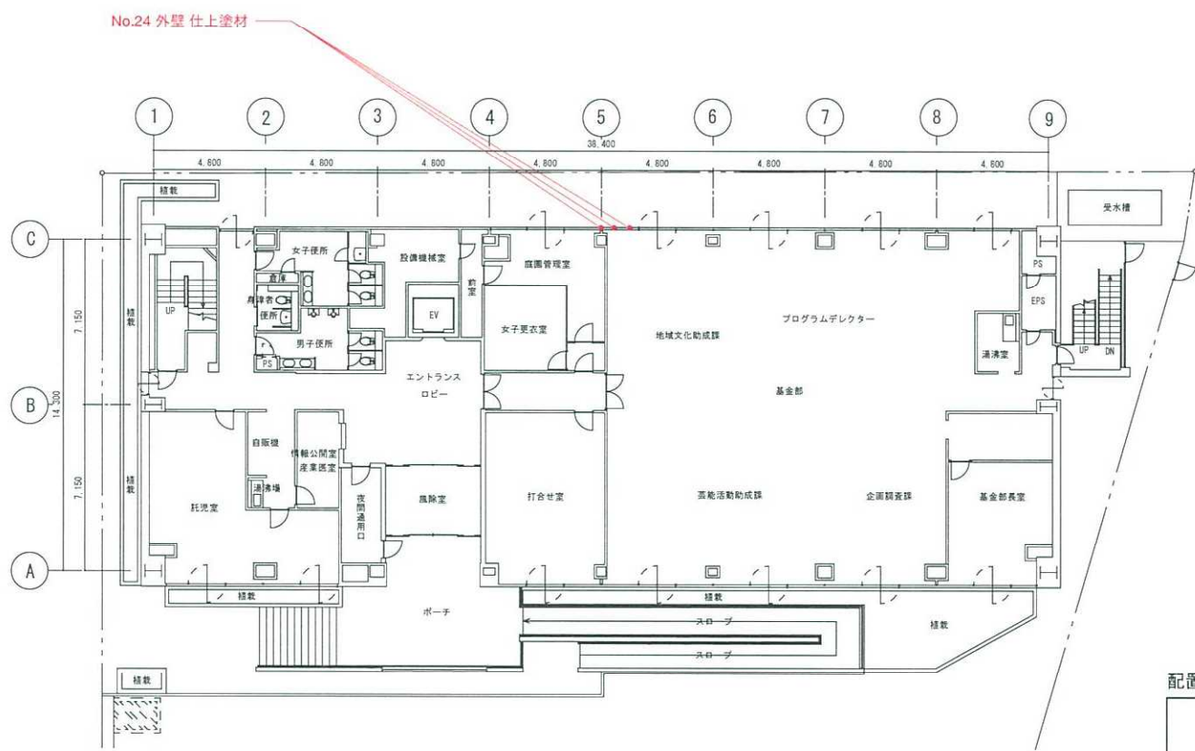
1階 平面図
