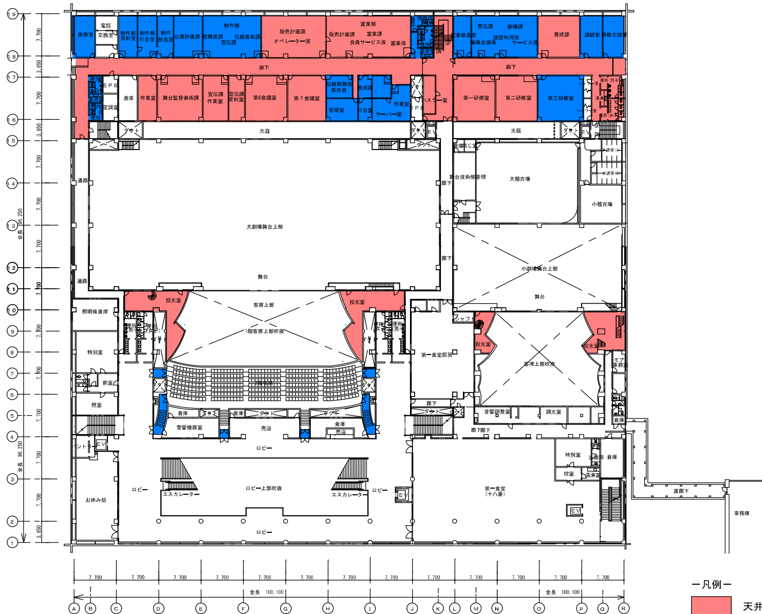
本館 2階平面図 S=1:500
