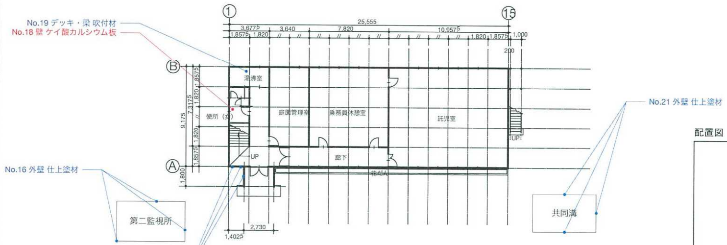
1階 平面図
