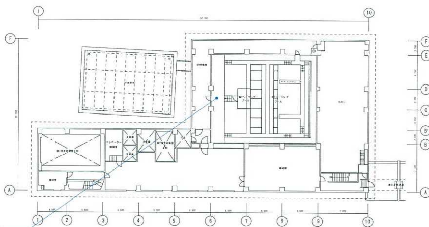
4階 平面図
