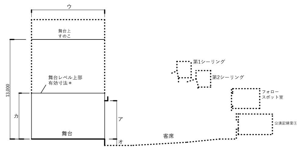
断面図
