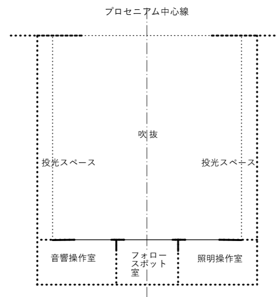
第二層平面図
