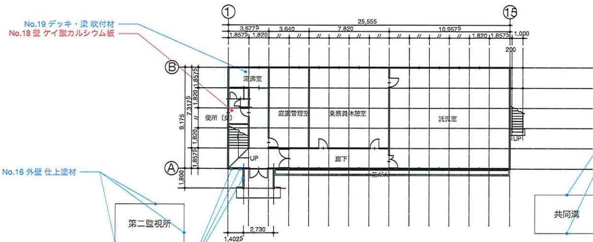
1階 平面図
