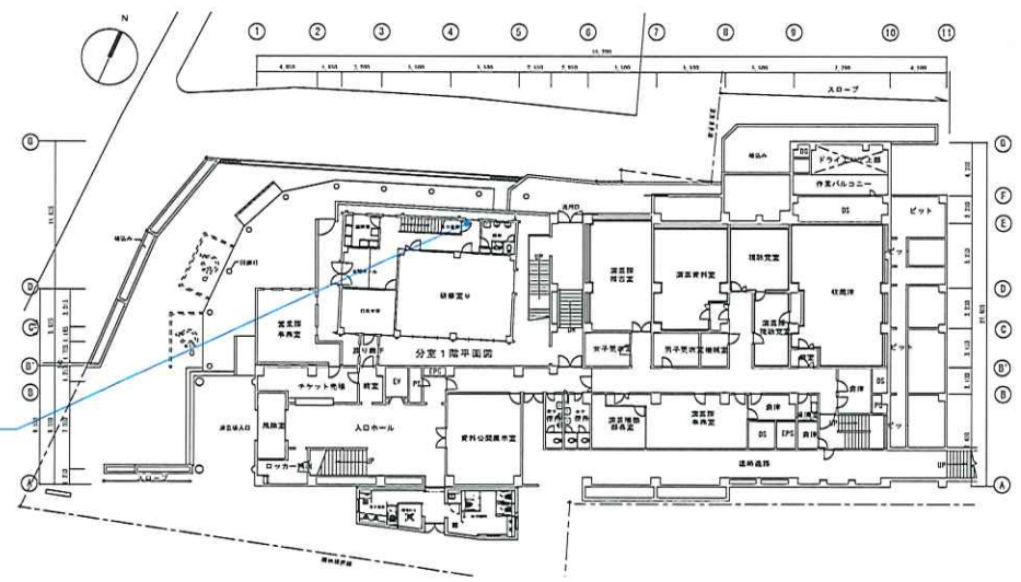
1階 平面図
