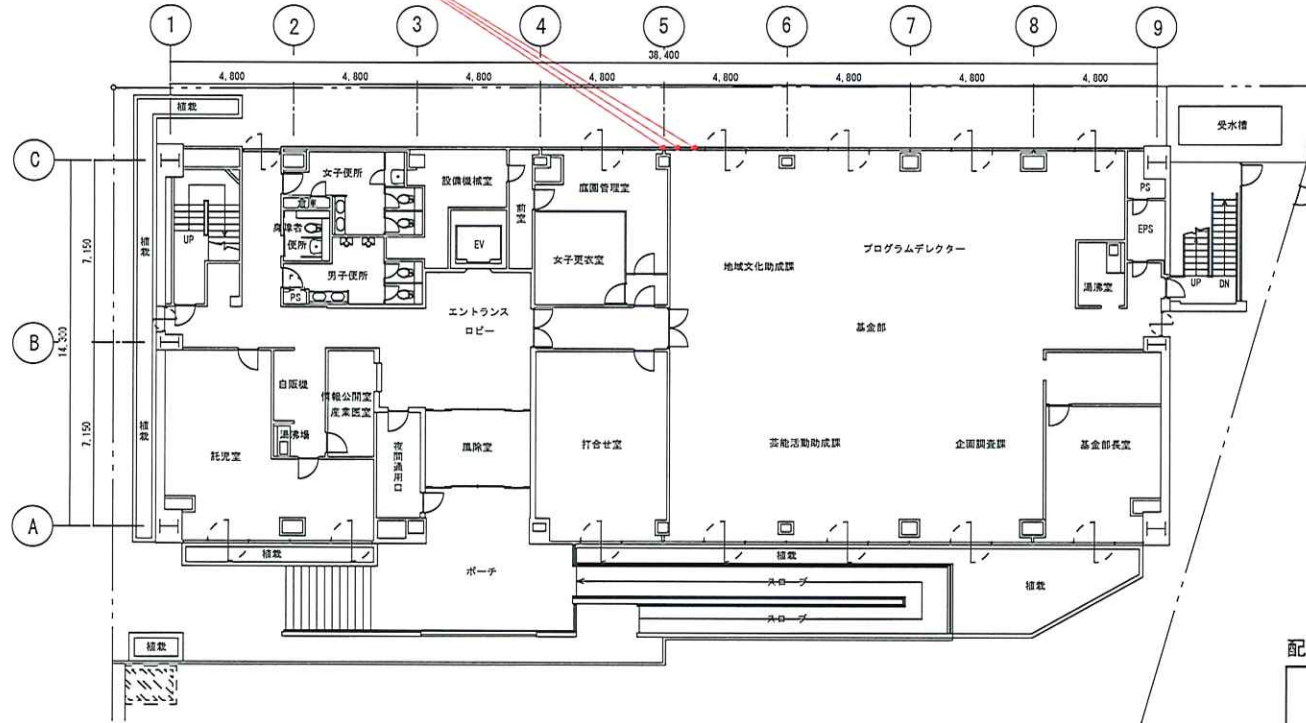
1階 平面図
