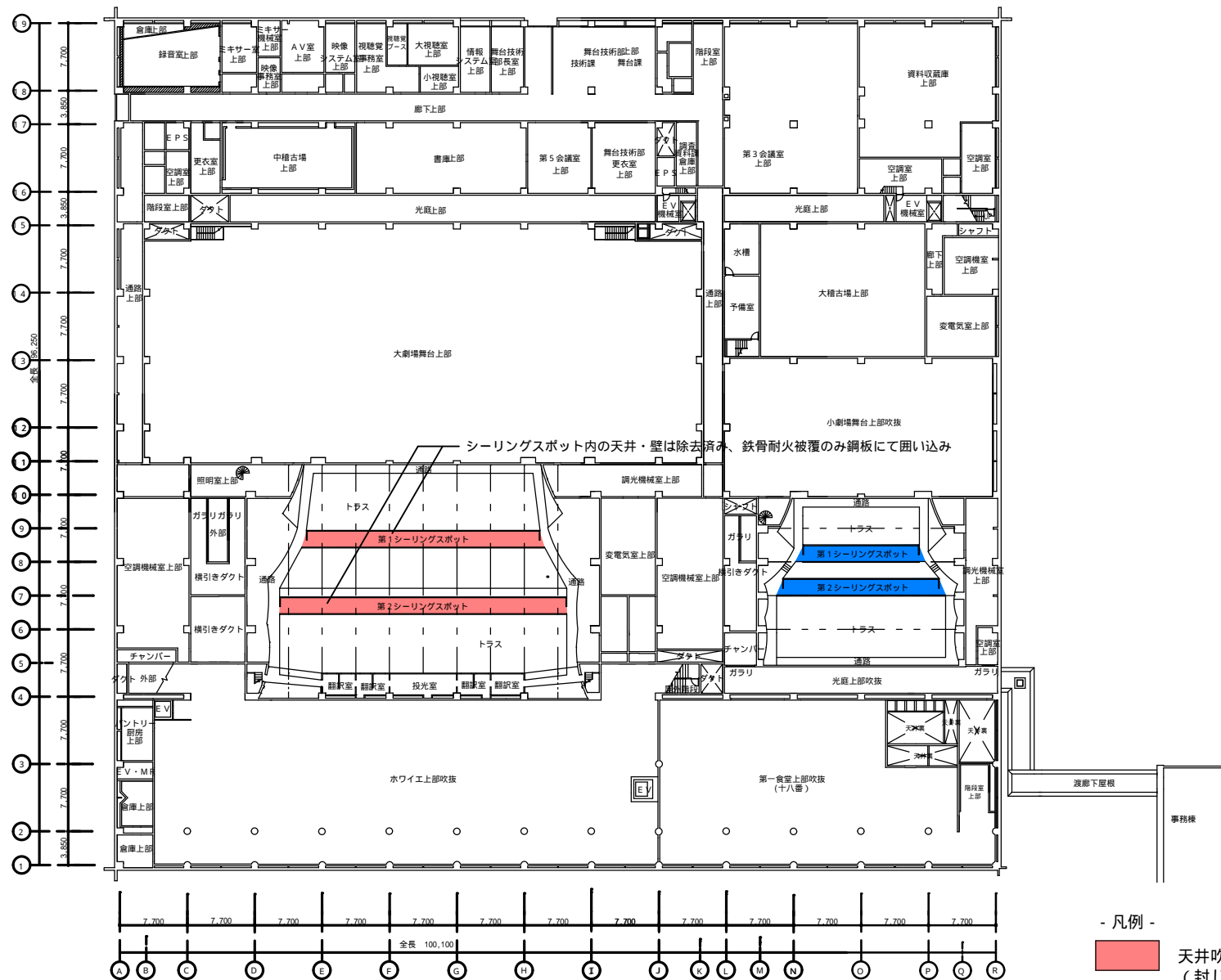
本館 3階上部平面図 S = 1 : 5 0 0
