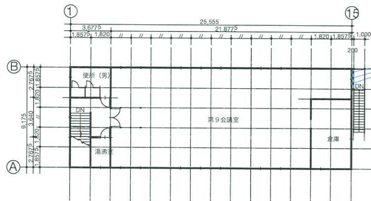
2階 平面図
