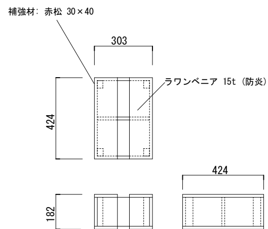
箱馬(1.4 × 1.0 × 0.6) 424 × 303 × 182
