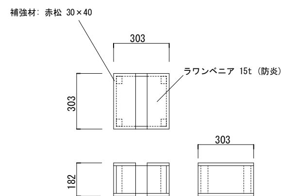
箱馬(1.0 × 1.0 × 0.6) 303 × 303 × 182
