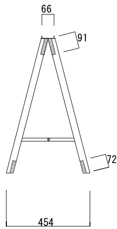
開き足(高足・4尺) 1,212×730 開き足(高足)
