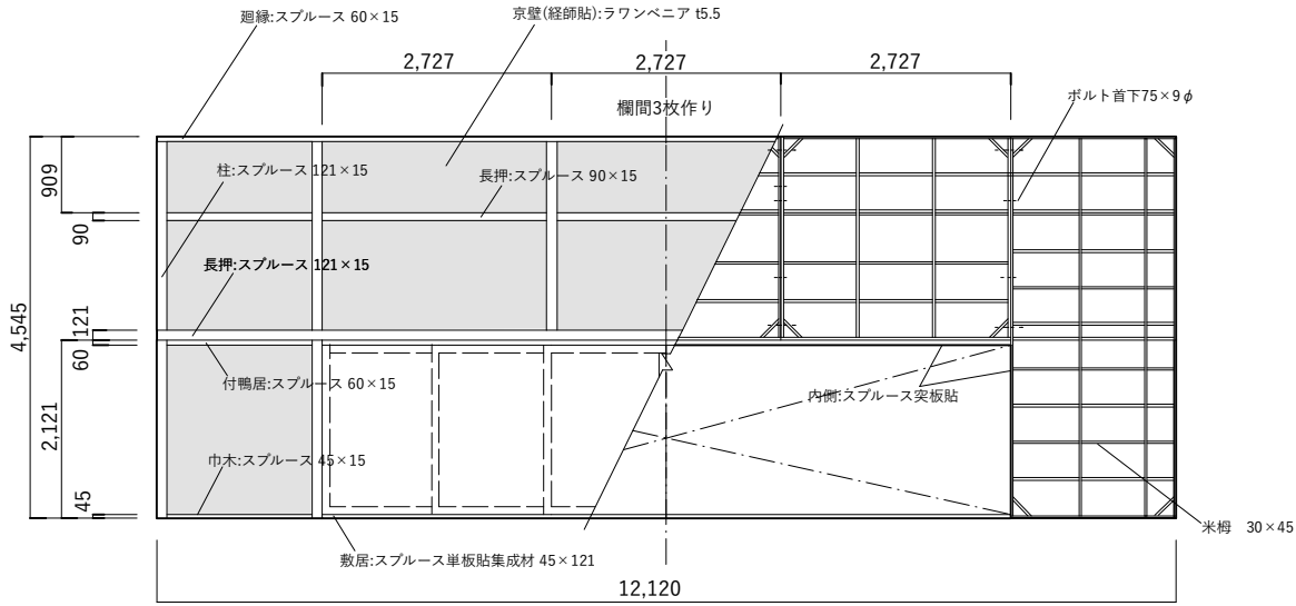
Ⓐ 大平 立面図/構造図
