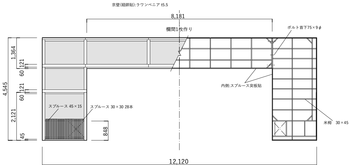
Ⓓ 前欄間 立面図/構造図
