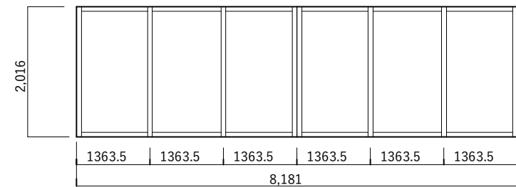
Ⓔ 6枚組板戸(襖)
