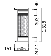
Ⓒ' 立面図
