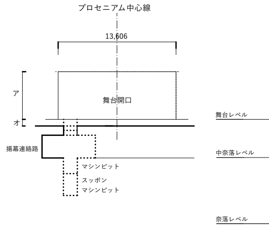
客席断面図
