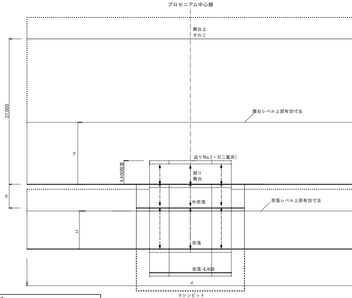
舞台断面図
