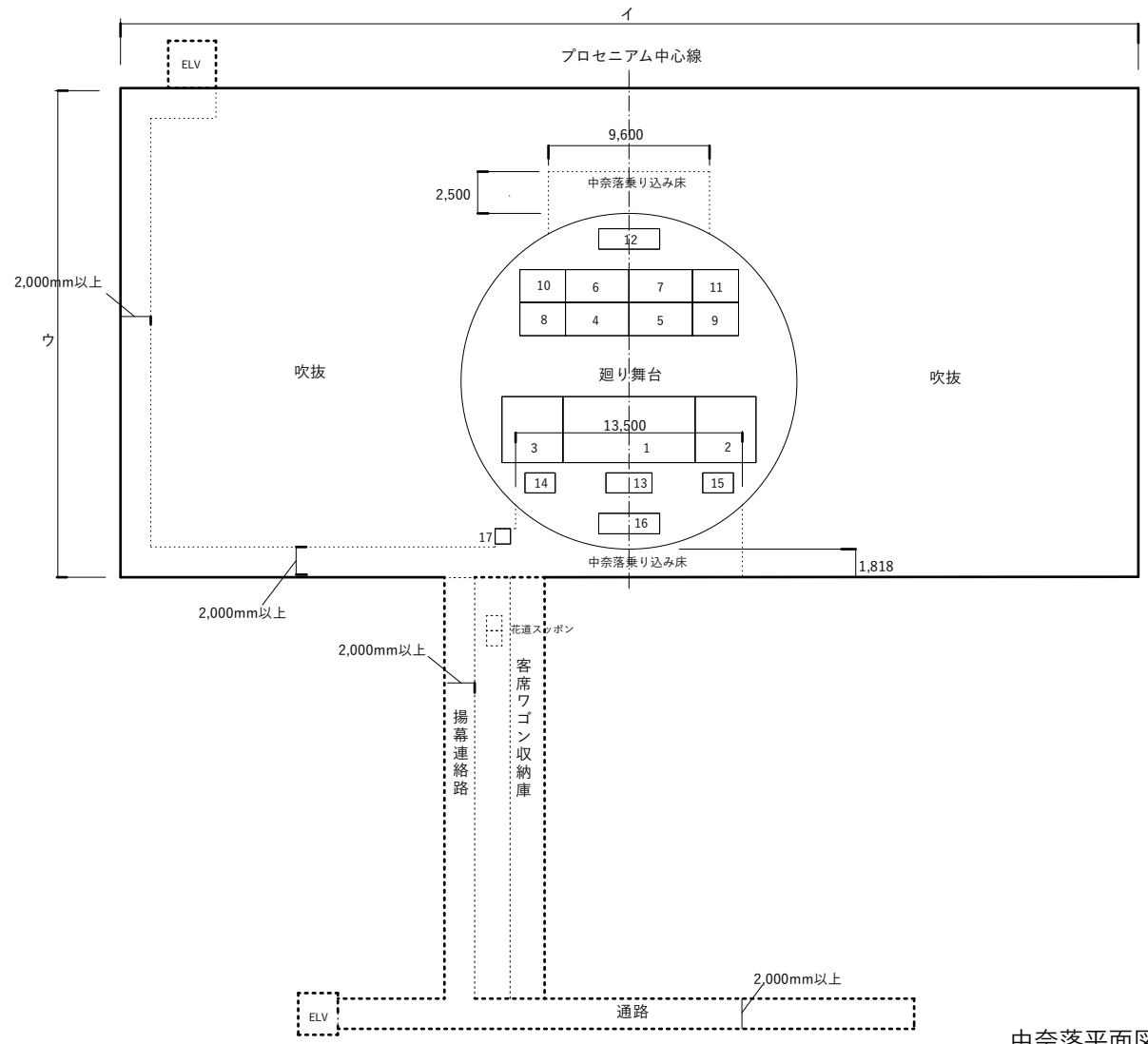
中奈落平面図
