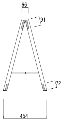
開き足(高足) 1,212×730 開き足(高足)
