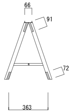
開き足(中足) 1,212×518 開き足(中足)
