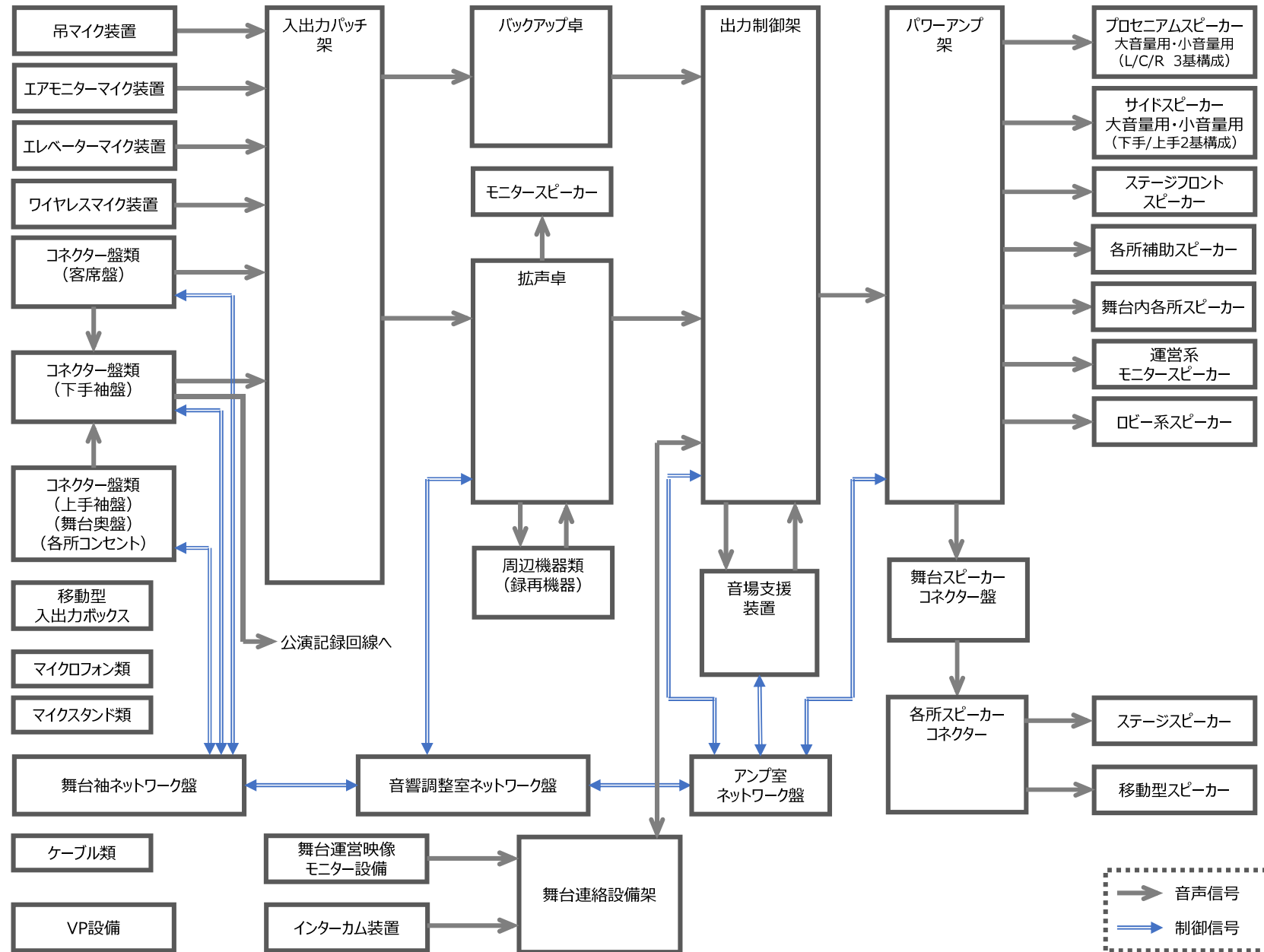
国立劇場 演芸場 舞台音響設備 ブロック系統図
