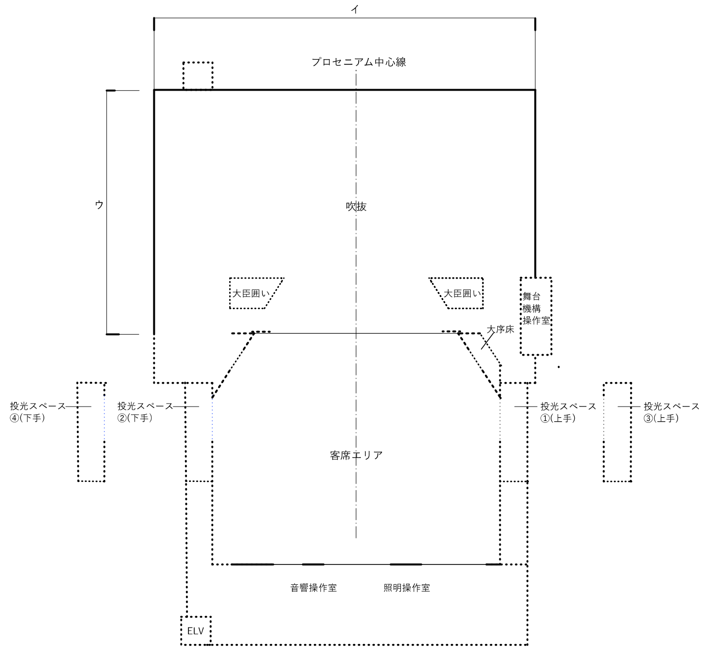
第二層平面図
