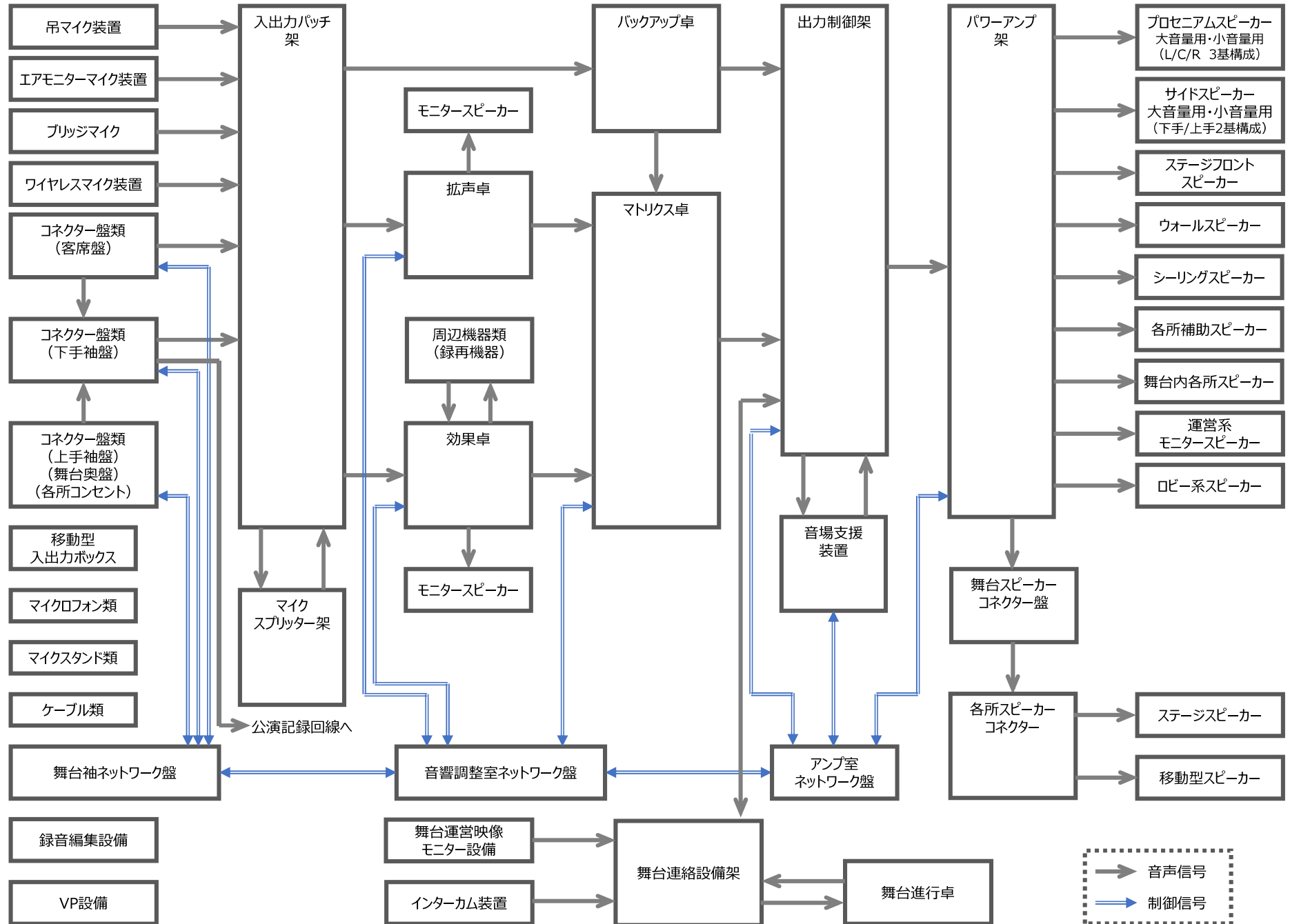
国立劇場 大劇場 舞台音響設備 ブロック系統図
