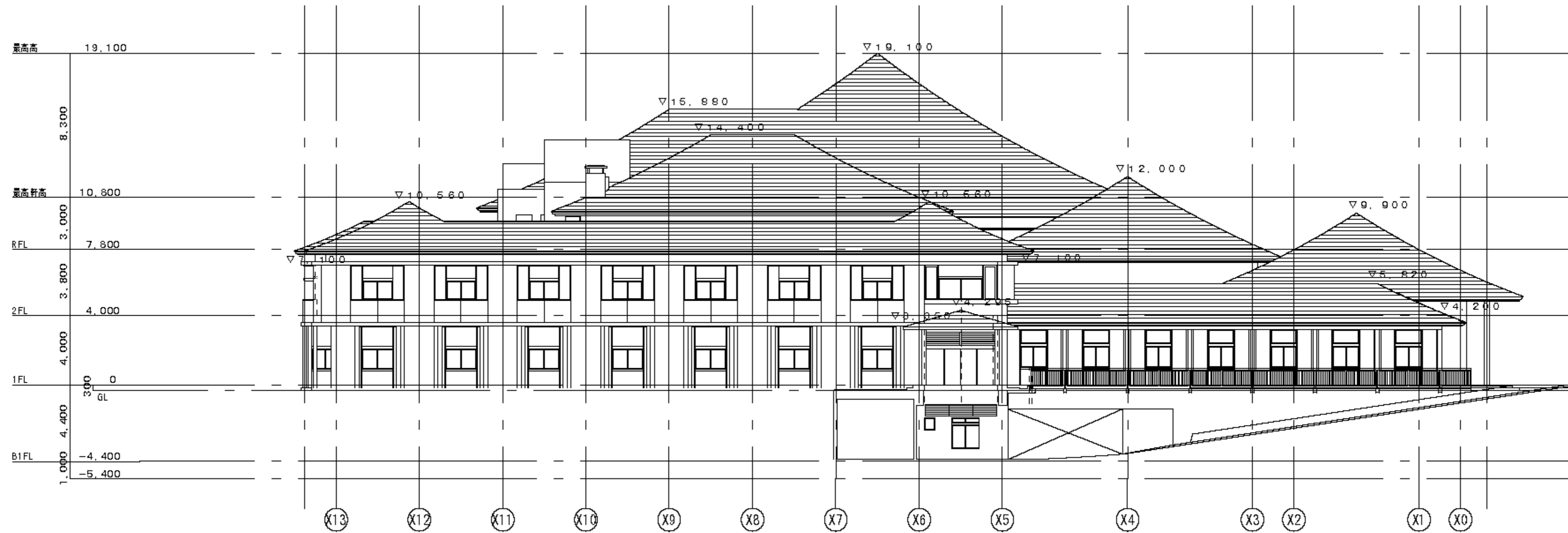
北側立面図 S=1/400
