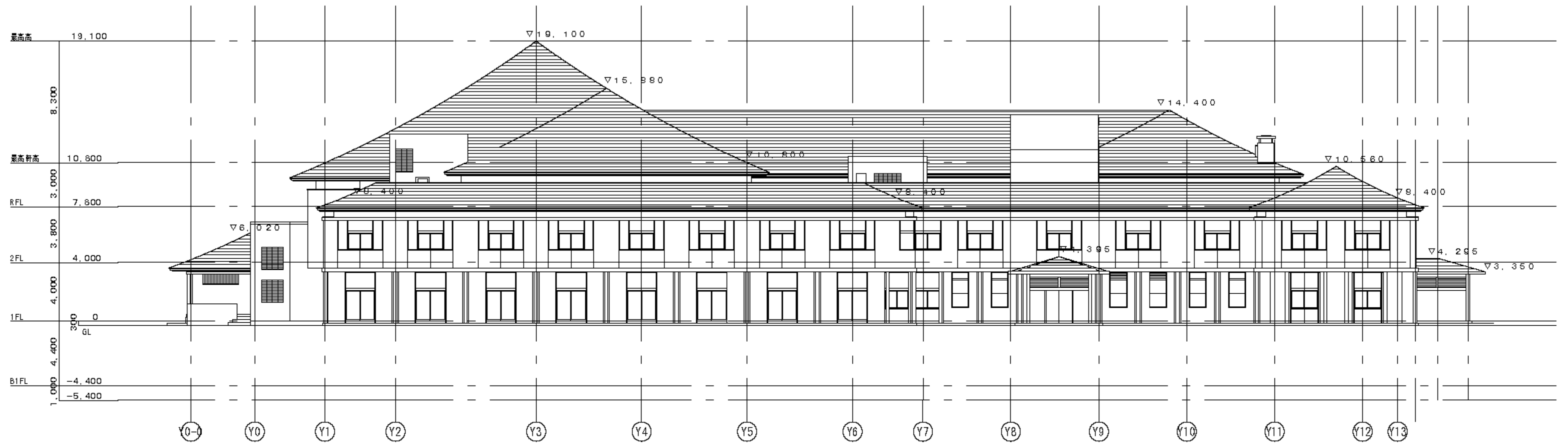
东侧立面图 S=1/400
