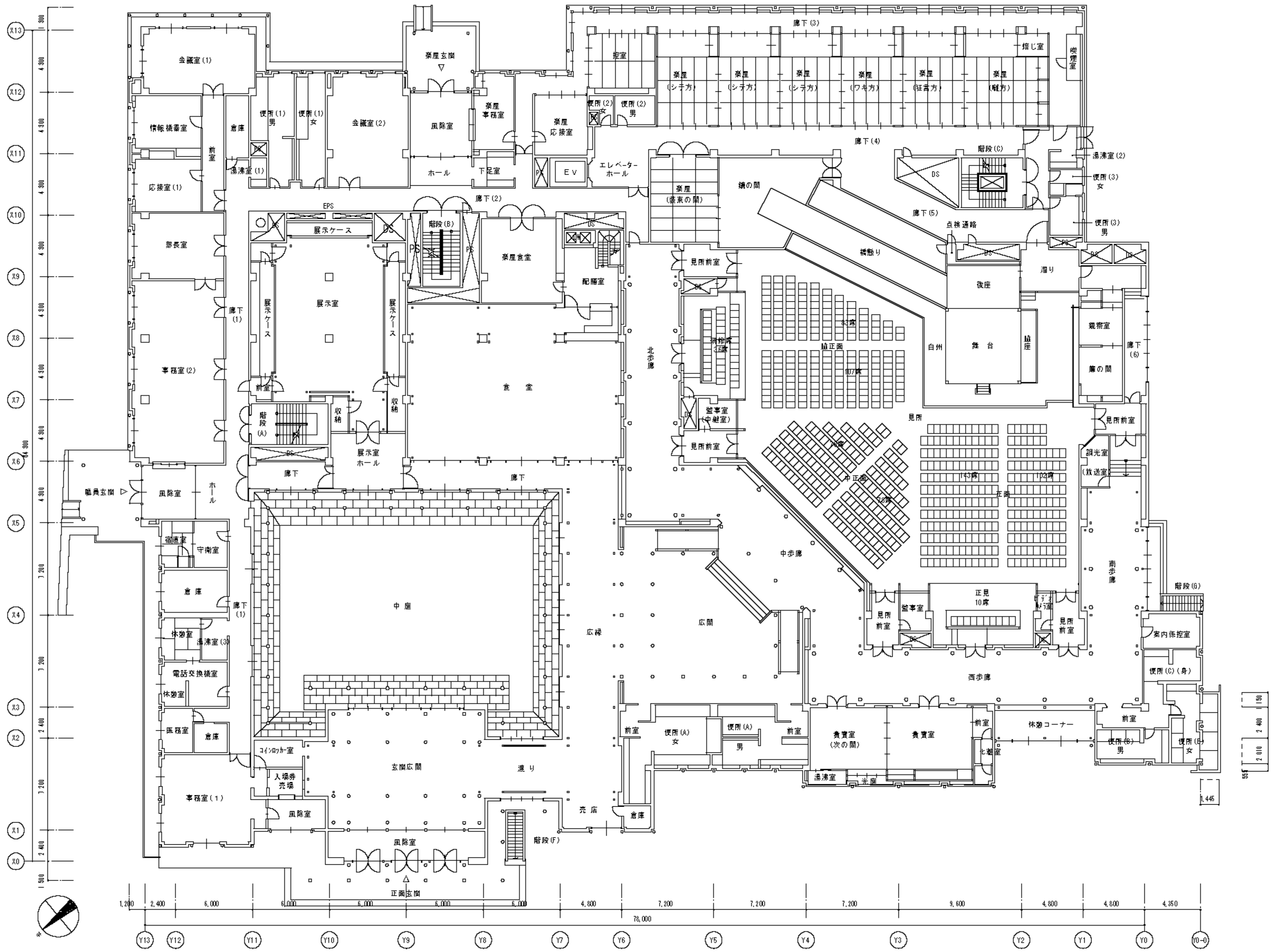
1階平面図 S=1/300
