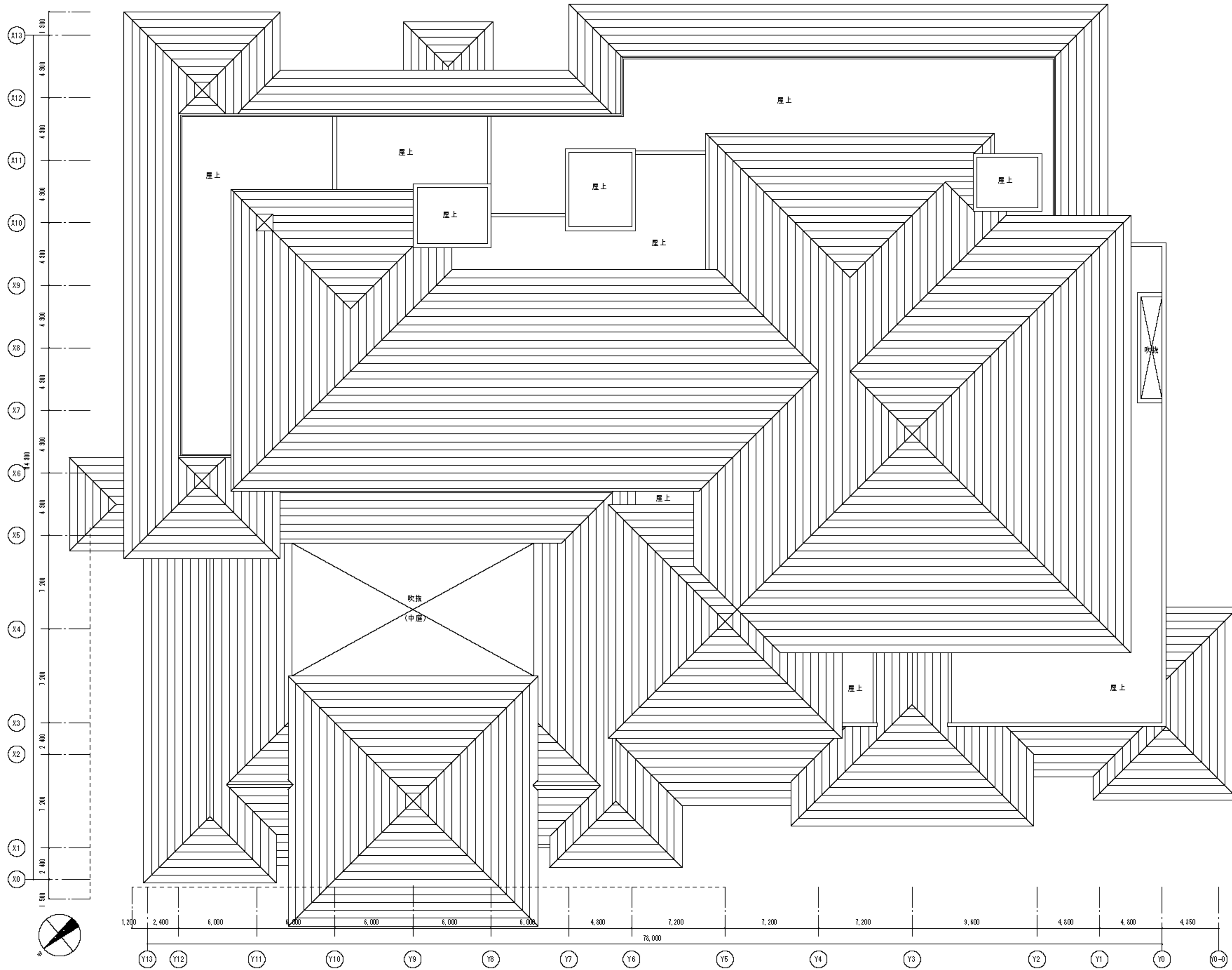
屋根伏図 S=1/300
