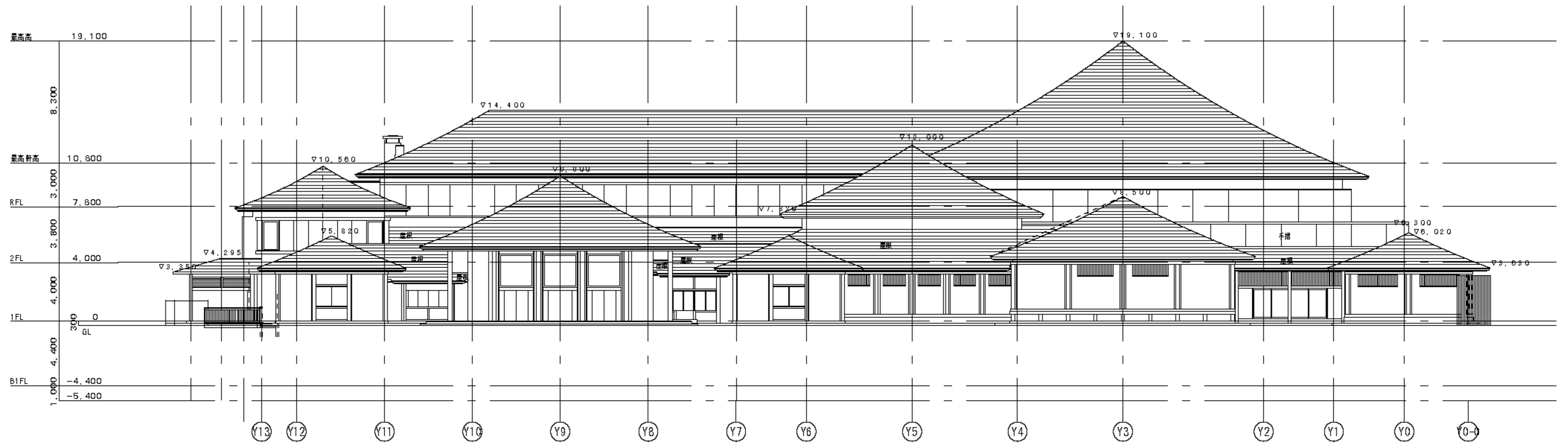
西側立面図 S=1/400
