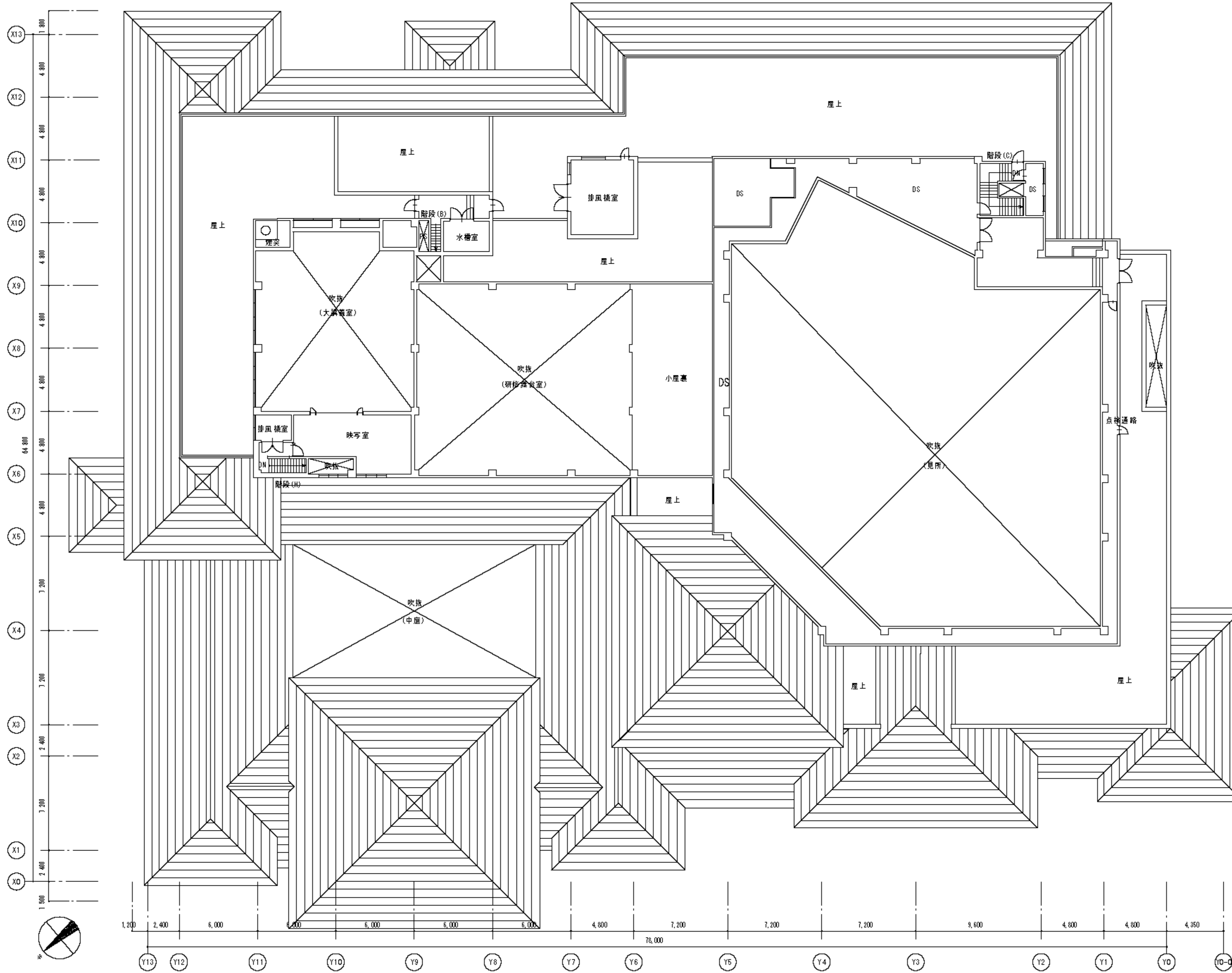
屋上平面圖 S=1/300
