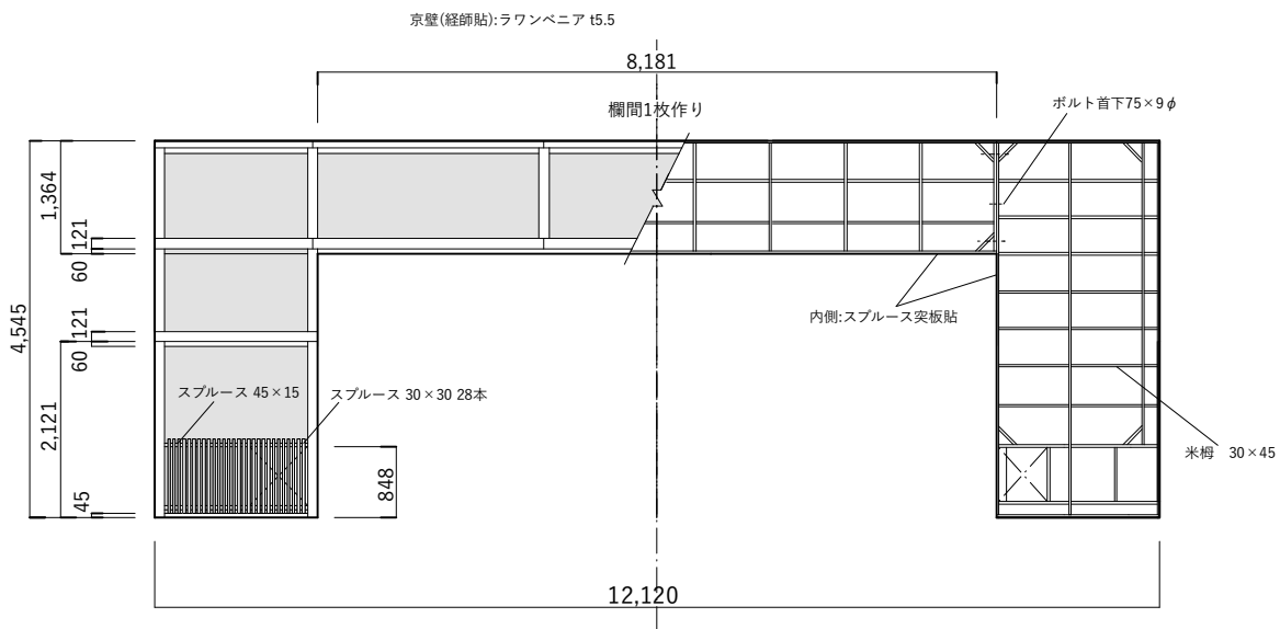
Ⓓ 前欄間 立面図/構造図
