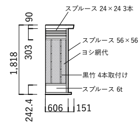
Ⓒ 立面図
