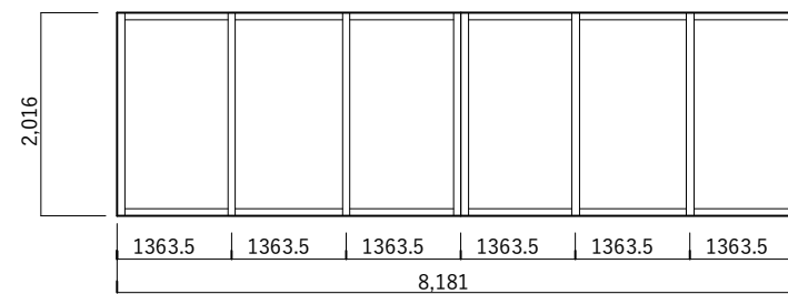
Ⓔ 6枚組板戸(襖)
