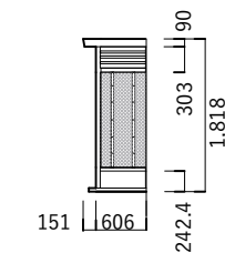
Ⓒ' 立面図
